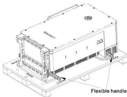
Obr. 5.8 Schéma zvedání
