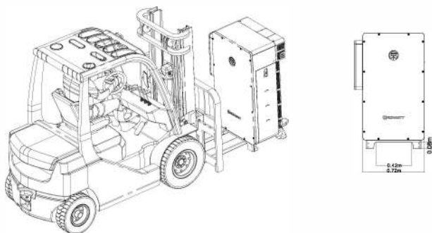
Obr 5.7 manipulace se střídačem za pomoci vysokozdvizného vozíku
