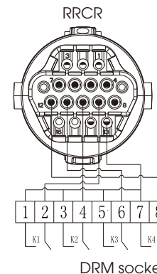
Obr. 6.20 střídač - RRCR připojení
