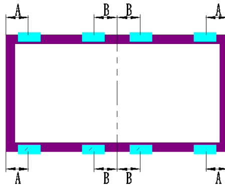
Použijte 8 svorek na dlouhé straně.
